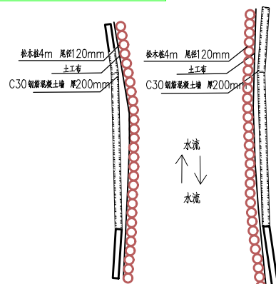
桥两边围堰大样图
