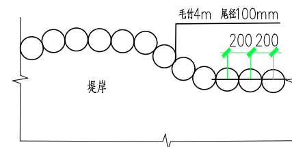
毛竹护堤大样图
