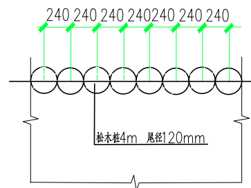
松木桩护堤大样图
