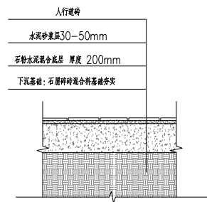
路面恢复基础大样图
