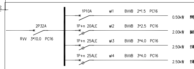
配电系统图 1:50
