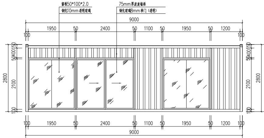
A立面图 1:50
