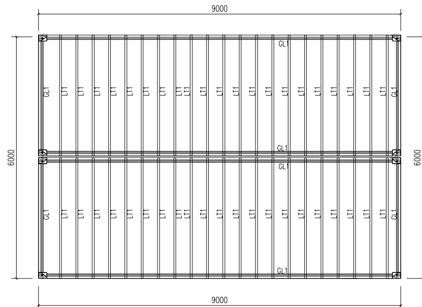
底座钢构布置图 1:50
