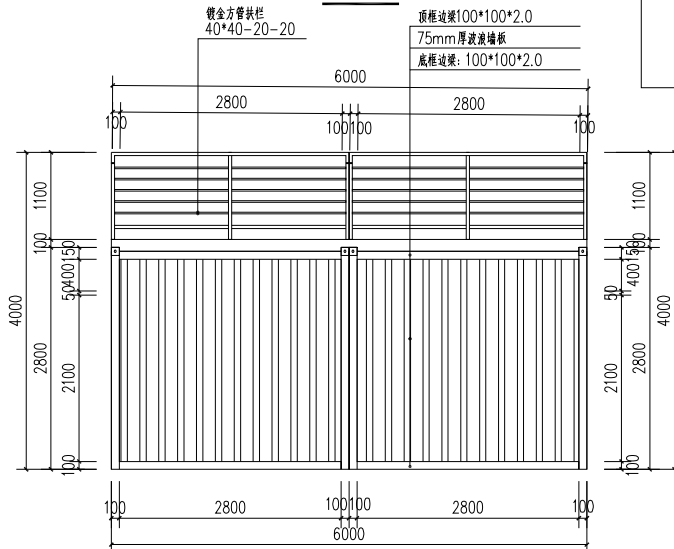
D立面图 1:50
