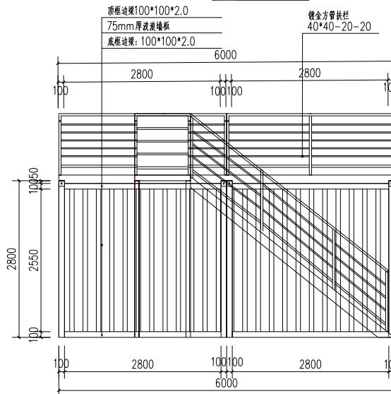
B立面图 1:50
