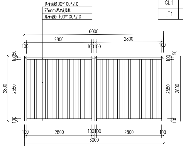
B立面图 1:50
