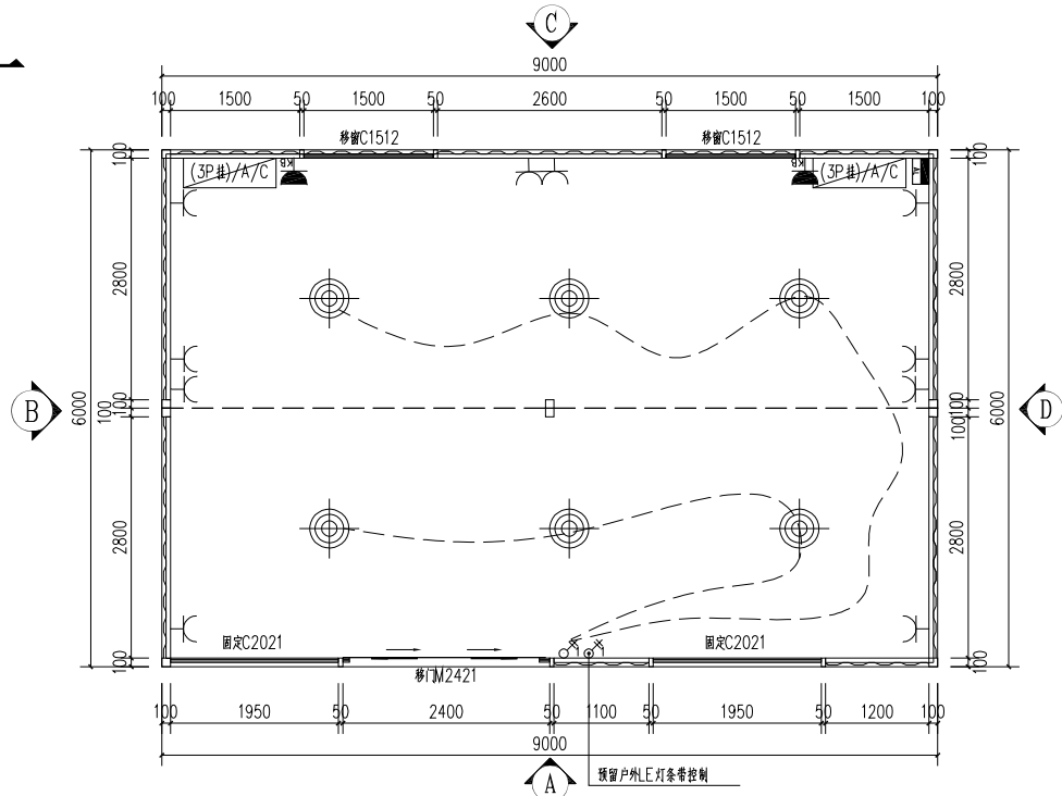
平面图 1:50
