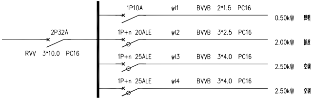
配电系统图 1:50
