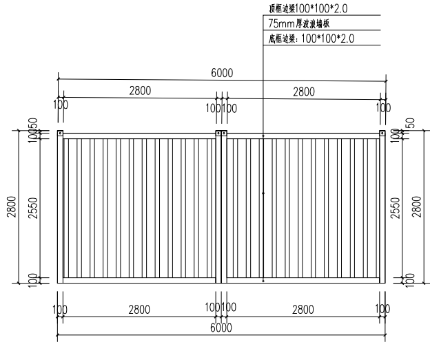
D立面图 1:50
